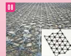
テンサー® TX 路盤補強工法用 三軸ジオグリッド
